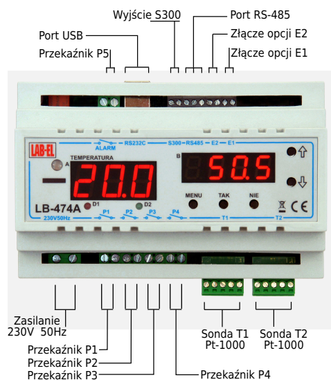
Figure 1: LB-474A3 – punkty wejść i wyjść
